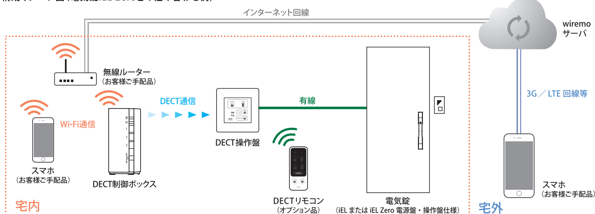
構成イメージ図 (電気錠 iEL Zero との組み合わせ例)
